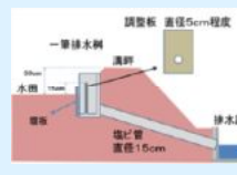
田んぼダムの概要
